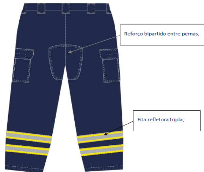
Figura 4: Desenho da Calça - Tardoz
